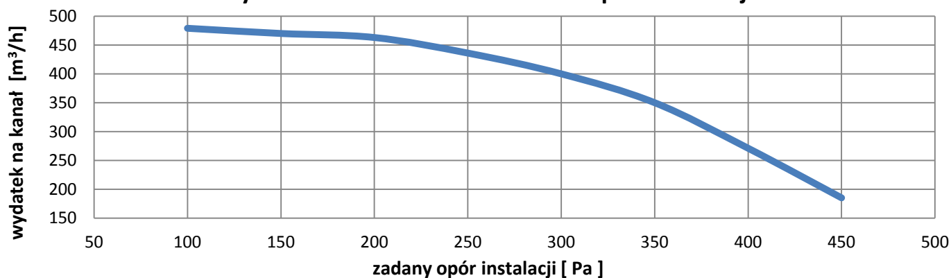
wydatek na kanał w zależności od oporu instalacji
