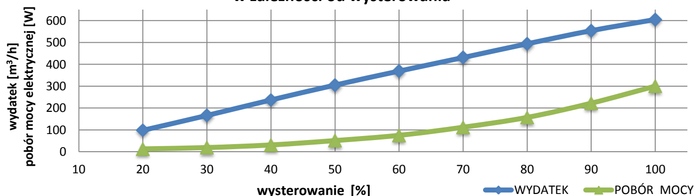
wydajność i pobór mocy elektrycznej w zależności od wysterowania
