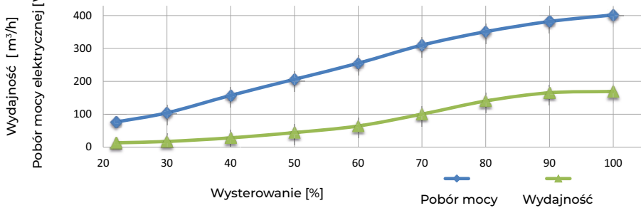
Wydajność i pobór mocy elektrycznej w zależności odysterowania
