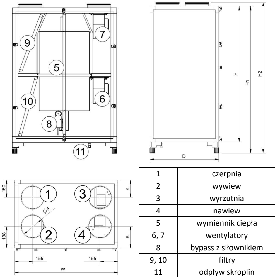
Rys. 1* Schemat budowy centrali „G” z wyszczególnieniem części składowych.
